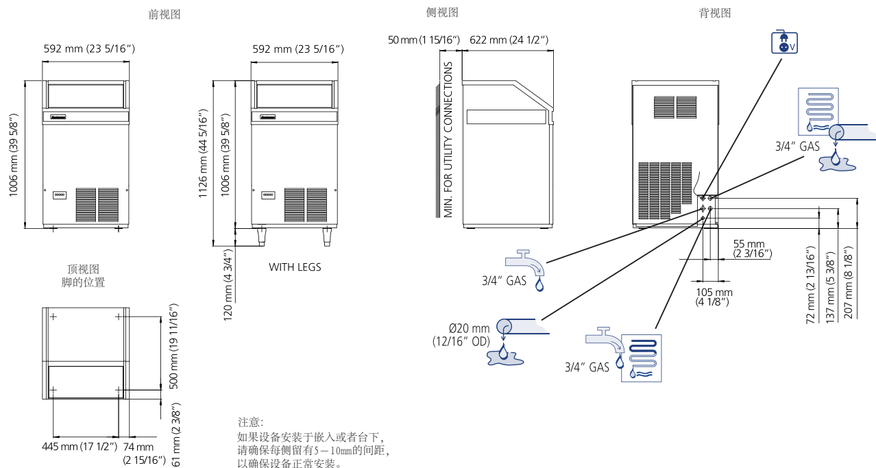
AF 103 风冷式
