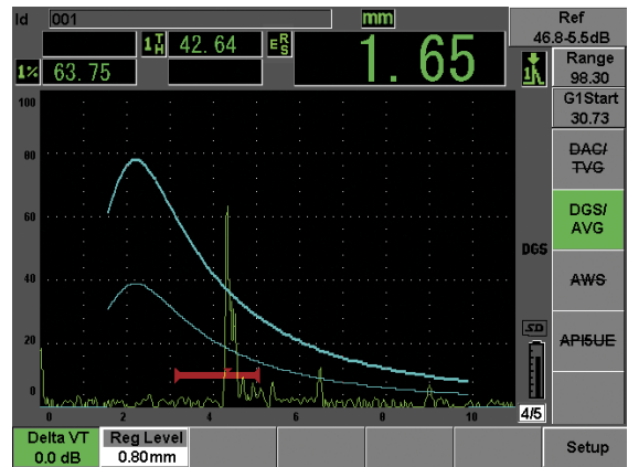
EPOCH 600型仪器的动态DGS/AVG特性
